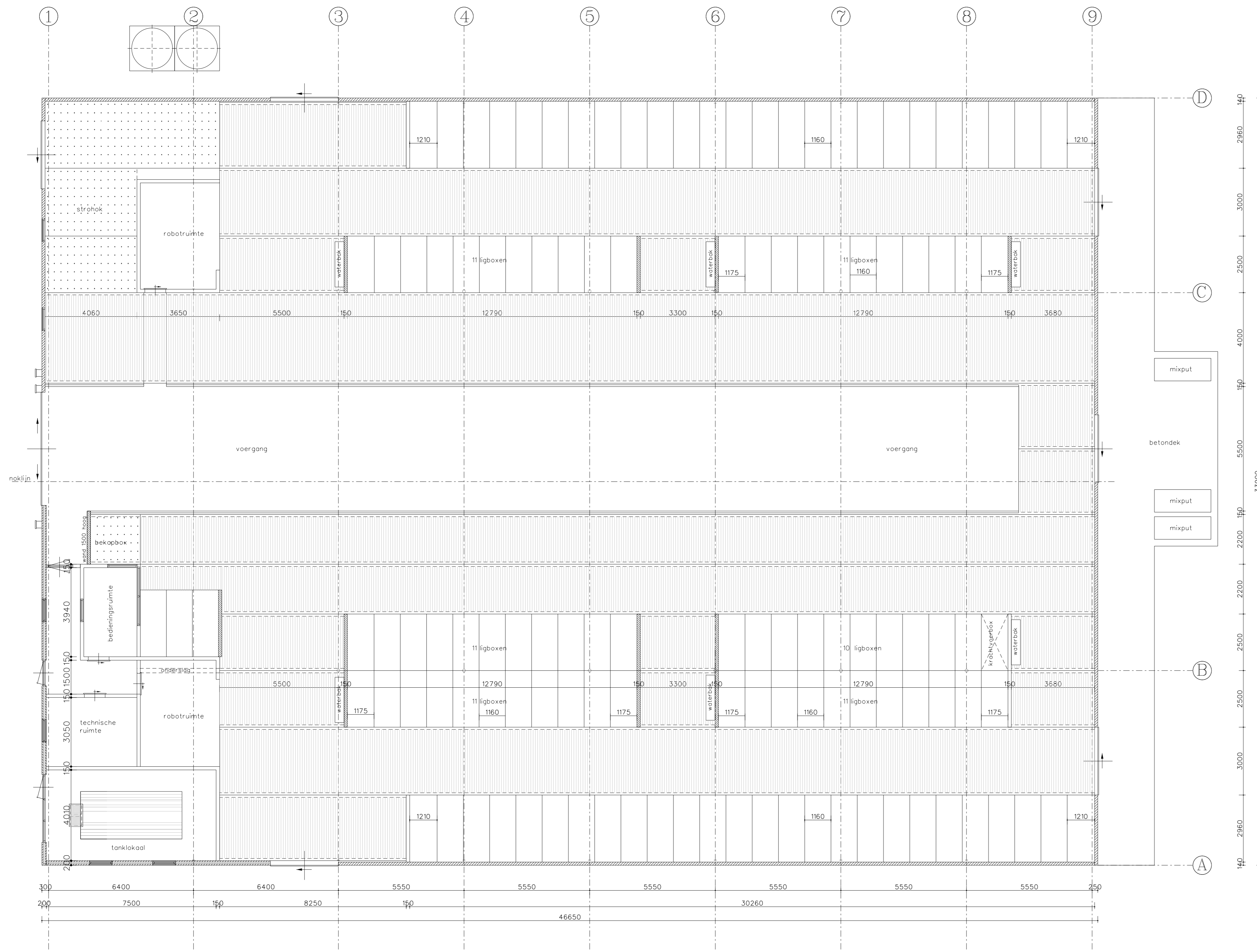
Plattegrond
