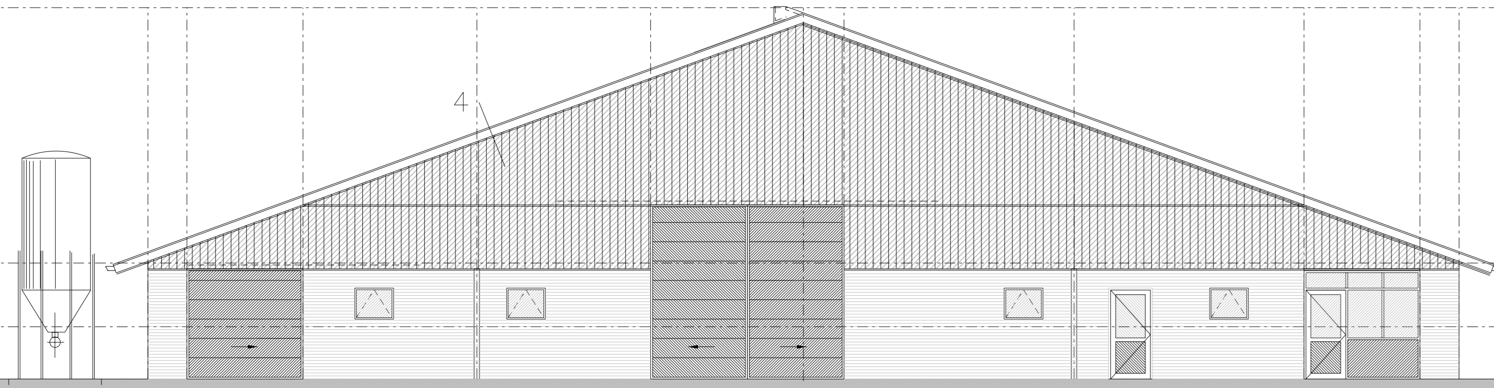
Voorgevel
