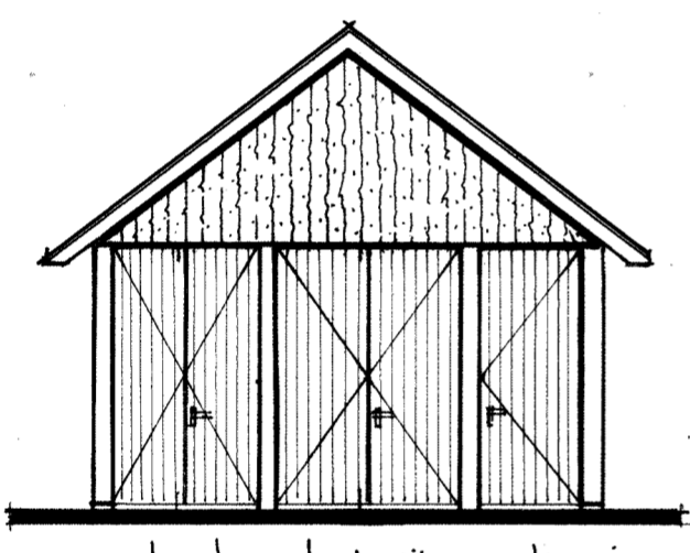
Voorgevel. deuren 15mm vrij van dorpel i.v.m ventilatie
