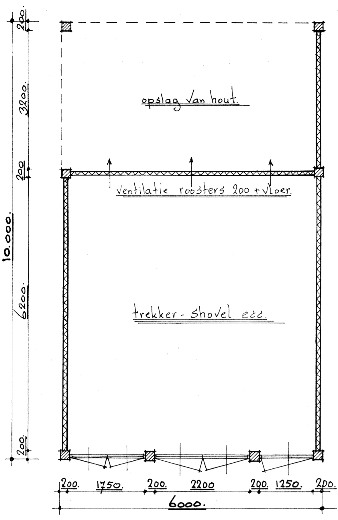
gebouw B. Schaal 1:50.
