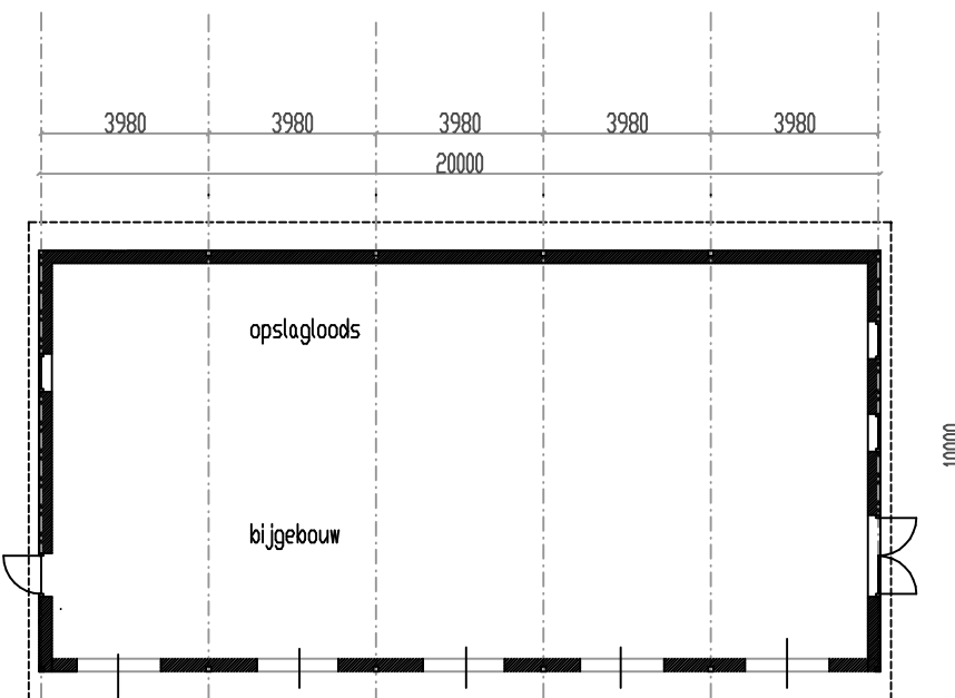
plattegrond
