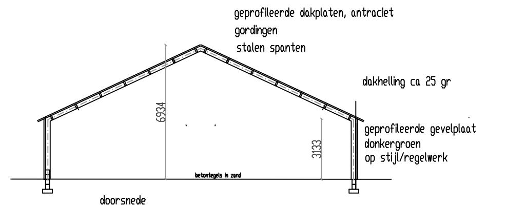
doorsnede
