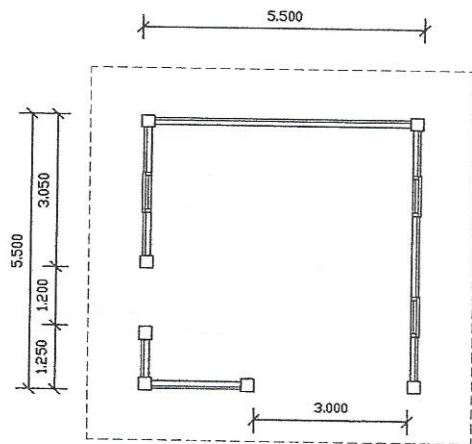
begane grond
