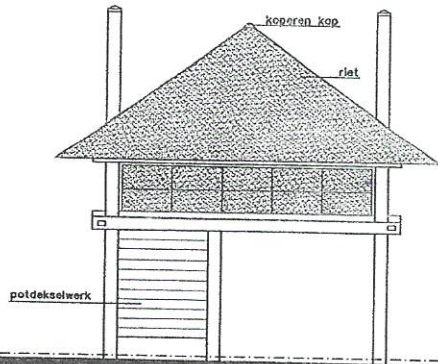
voorgevel
