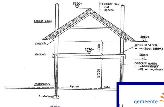
doorsnede
