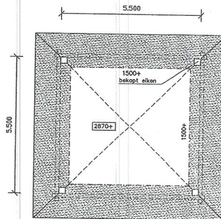
verdieping
