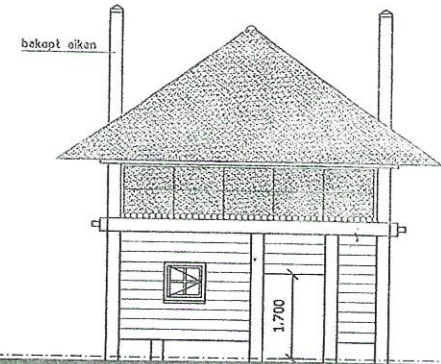
linkerzijgevel
