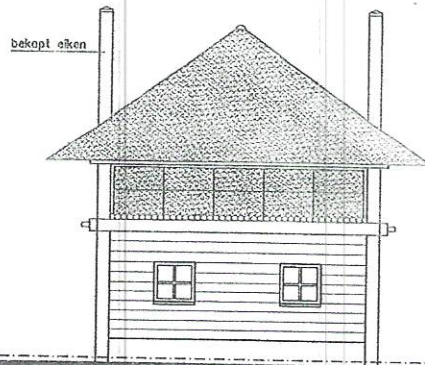
rechterzijgevel
