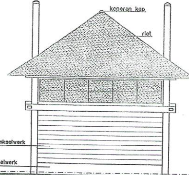
achtergevel
