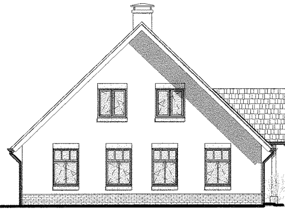
2 Linkerzij Gevel 1 : 100
