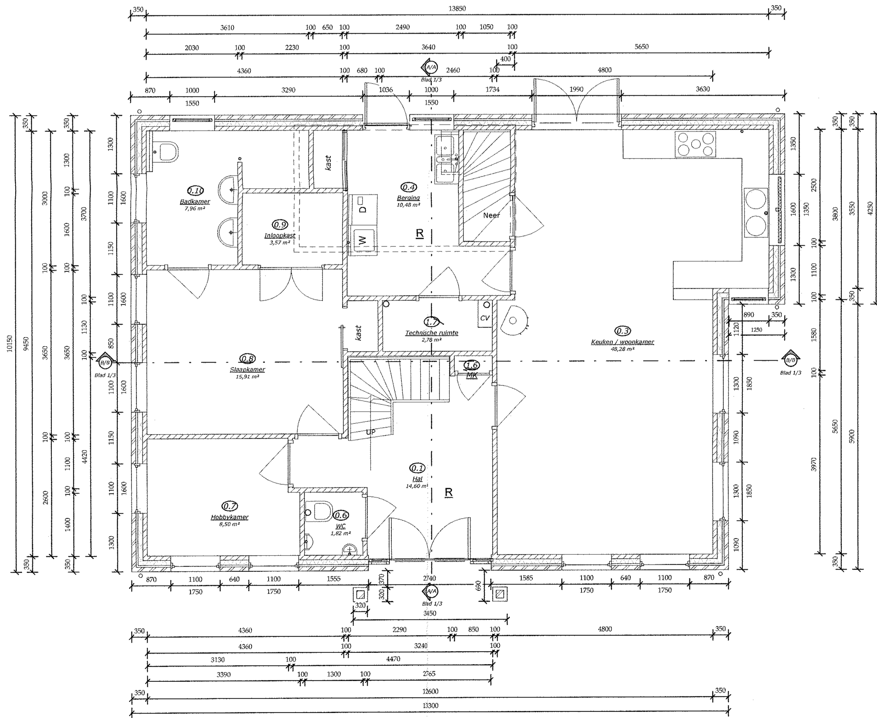
6 Begane Grond 1 : 50
