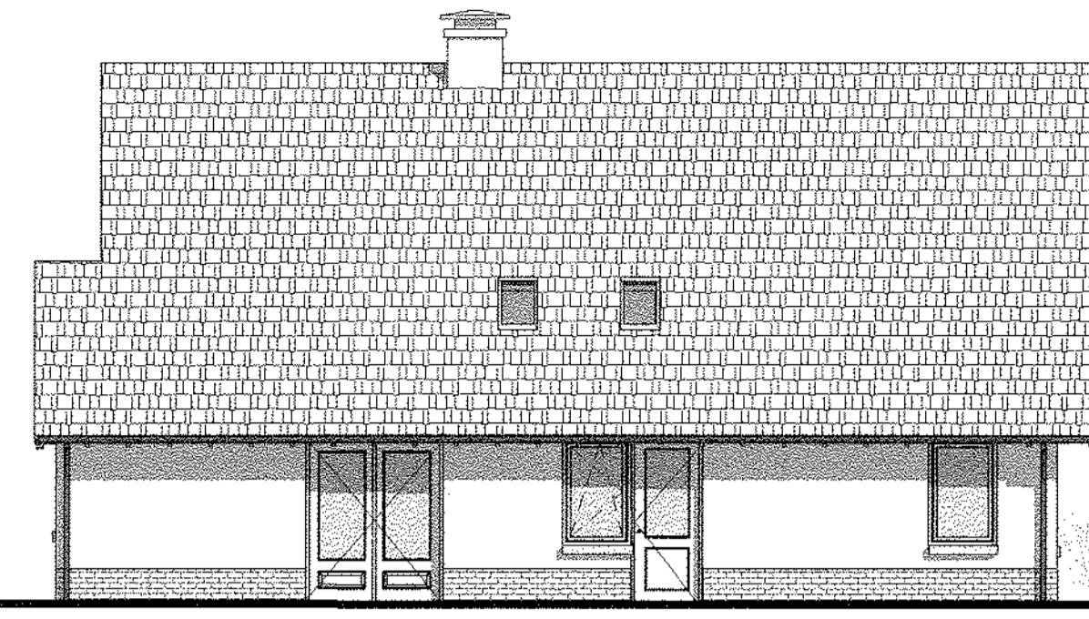
4 Achter Gevel 1 : 100
