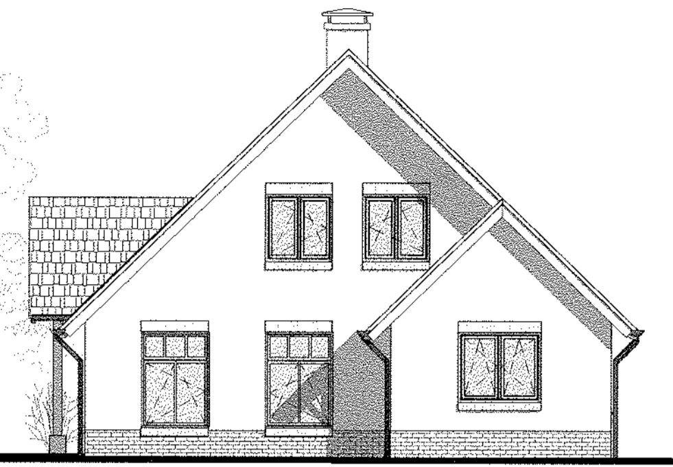
5 Rechterzij Gevel 1 : 100
