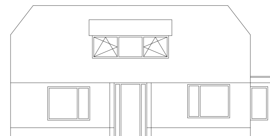
Rechterzijgevel gewijzigd
