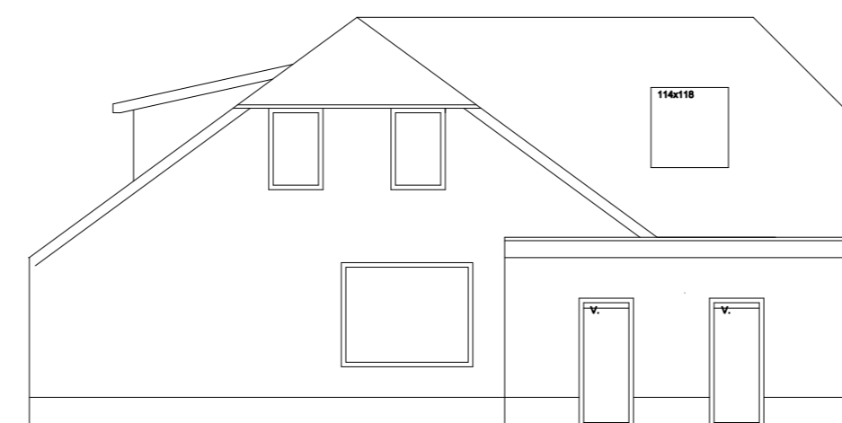
Achtergevel gewijzigd
