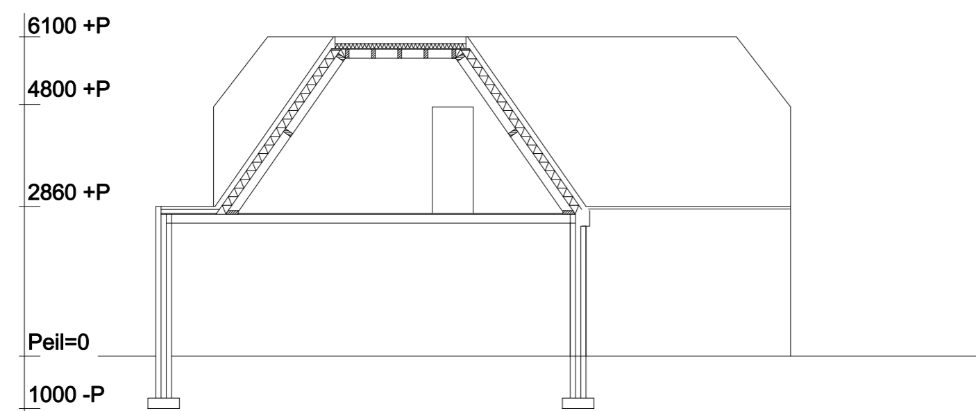
Doorsnede A-A
