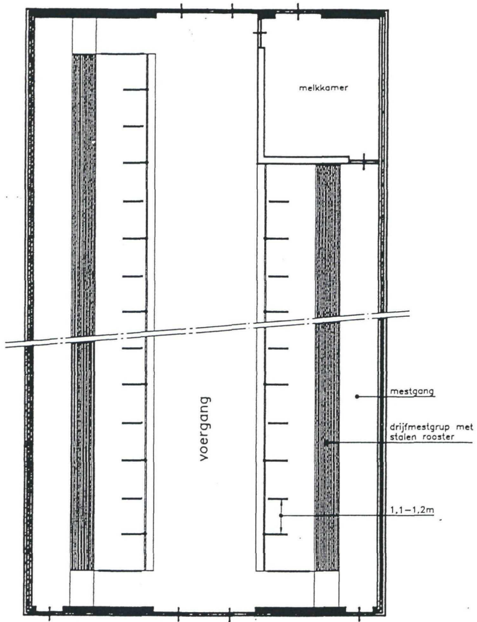
Plattegrond
