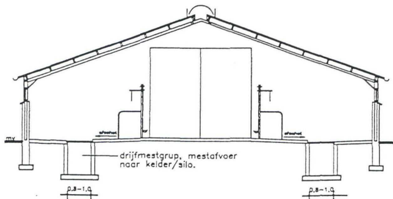
Dwarsdoorsnede
