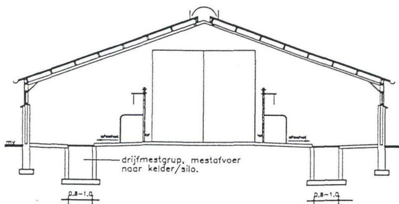
Dwarsdoorsnede
