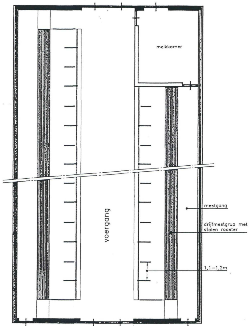
Plattegrond
