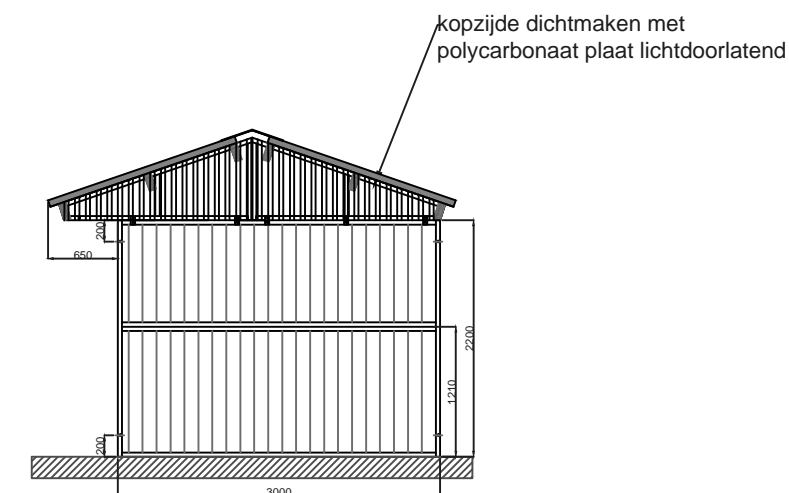
Aanzicht rechterzijde
