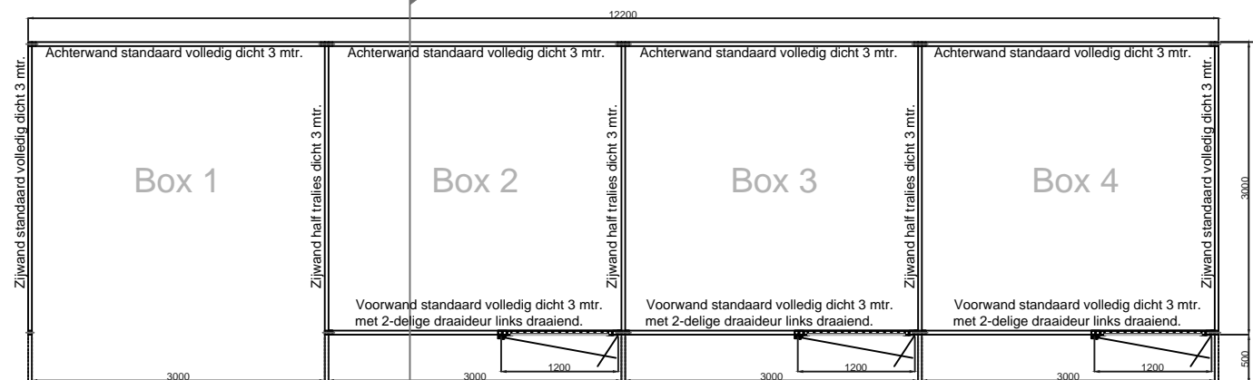
Plattegrond
