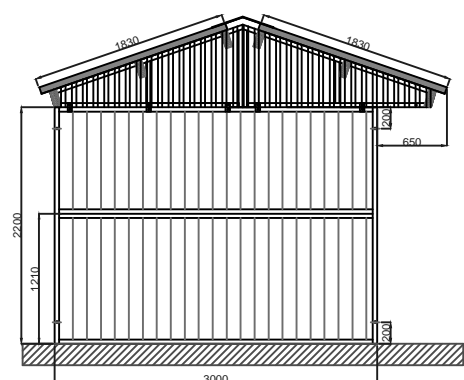
Aanzicht linkerzijde
