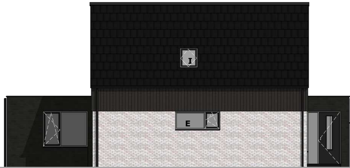
C LINKERZIJGEVEL / Noord-West A
